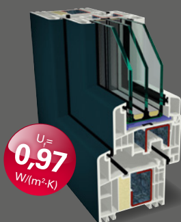
Telaio ed anta più alti in colorato
