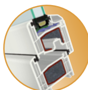
Sistema con anta complanare a 5 camere
