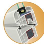
Sistema S 8000 IQ semicomplanare
